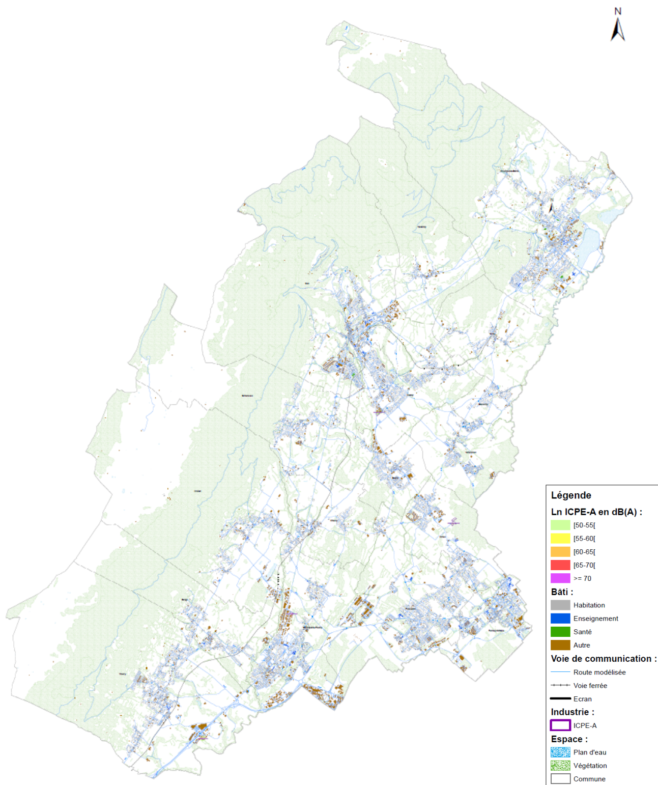
Exemple de carte du bruit industriel pour l'indicateur nocturne L_n
