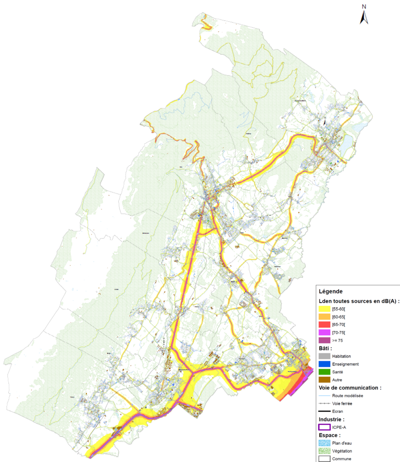
Exemple de carte de l'ensemble des sources de bruit pour l'indicateur global L_{den}
