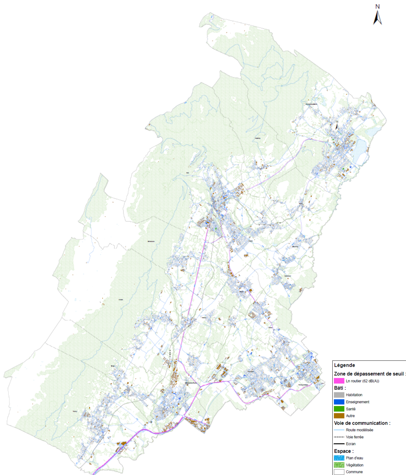
Exemple de carte des zones de dépassement de seuil du bruit routier pour l'indicateur nocturne L_n
